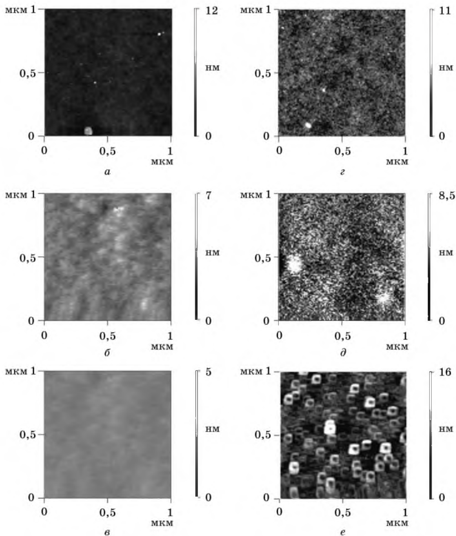
Рис. 2. АСМ-изображение поверхности золь-гель пленок, содержащих соединения Fe_xCo_yO_z - SiO_2 : a, б, в — нелегированных, отожженных при температуре a — 200 °С, б — 500 °С, в — 750 °С; г, д, e — Fe—Co-содержащих, отожженных при температуре г — 200 °С, д — 500 °С, e — 750 °С
