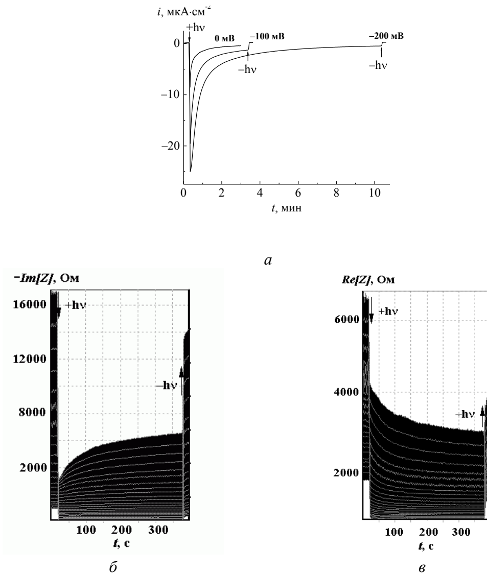
Рис. 3. Изменение тока при включении и выключении освещения на Se электроде в растворе 0,05 \text{ M CdSO}_4 + 0,05 \text{ M H}_2\text{SO}_4 + 1 \text{ M Na}_2\text{SO}_4 при разных значениях потенциала в области фотостимулируемого осаждения атомного слоя Cd (а) и кинетика изменения мнимого Im[Z] (б) и действительного Re[Z] (в) импеданса, измеренного на разных частотах, без освещения и при освещении. Каждая светлая линия на темном фоне соответствует импедансу на определенной частоте (б, в); частоты увеличиваются от 19 Гц до 702 Гц (сверху вниз)
