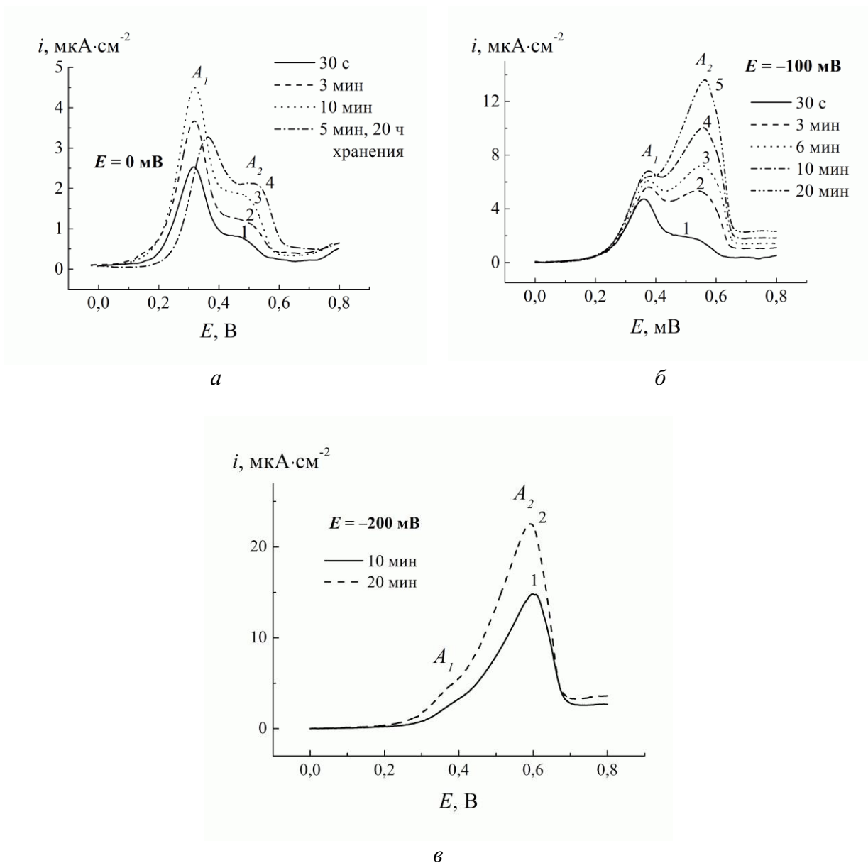
Рис. 4. Анодные потенциодинамические вольтамперограммы продуктов, полученных на Se-электроде в растворе 0,05 \text{ M CdSO}_4 + 0,05 \text{ M H}_2\text{SO}_4 + 1 \text{ M Na}_2\text{SO}_4 при облучении в течение разного времени при потенциалах, мВ: а — 0, б — -100, в — -200. dE/dt = 1,6 \text{ мВ/с}
