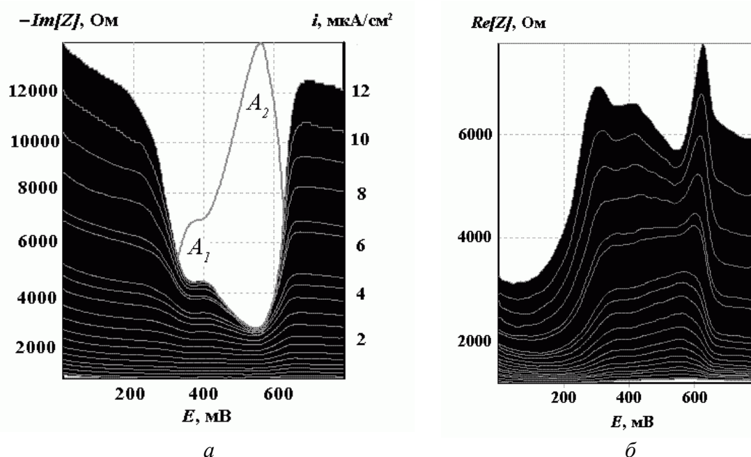
Рис. 5. Спектры ПДЭИС продуктов, полученных на Se-электроде в растворе 0,05 \text{ M CdSO}_4 + 0,05 \text{ M H}_2\text{SO}_4 + 1 \text{ M Na}_2\text{SO}_4 при облучении в течение 20 мин при потенциале -100 \text{ мВ} :
