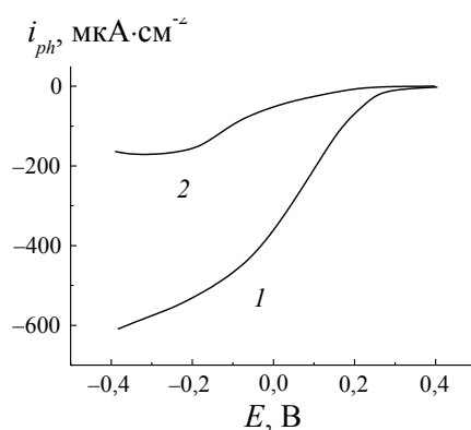
Рис. 2. Потенциодинамические кривые катодного фототока Se-электрода в растворах, содержащих и не содержащих \text{Cd}^{2+} : 1 – 0,05 М \text{H}_2\text{SO}_4 + 1 М \text{Na}_2\text{SO}_4 ; 2 – 0,05 М \text{CdSO}_4 + 0,05 М \text{H}_2\text{SO}_4 + 1 М \text{Na}_2\text{SO}_4
