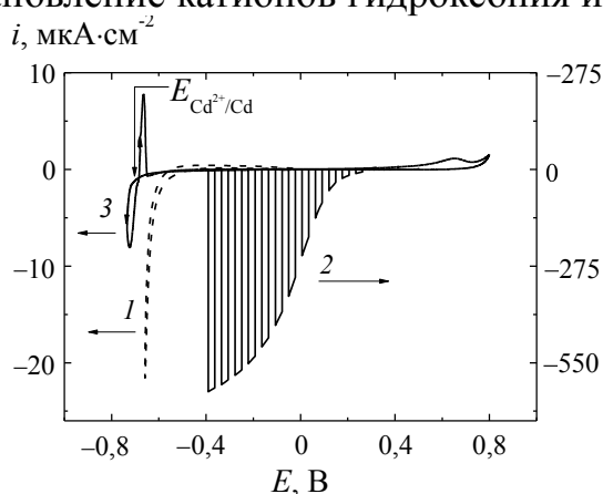
Рис. 1. Потенциодинамические поляризационные кривые для Se-электрода в растворах: 1, 2 – 0,05 М H_2SO_4 + 1 М Na_2SO_4 ; 3 – 0,05 М CdSO_4 + 0,05 М H_2SO_4 + 1 М Na_2SO_4 . Кривые 1, 3 записаны в темноте, а кривая 2 – при прерывистом освещении электрода белым светом
